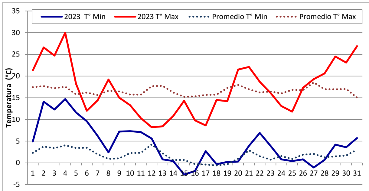
Gráfico 3. Línea de puntos: promedio histórico (2001-2023); Línea continua: registros año 2023.
