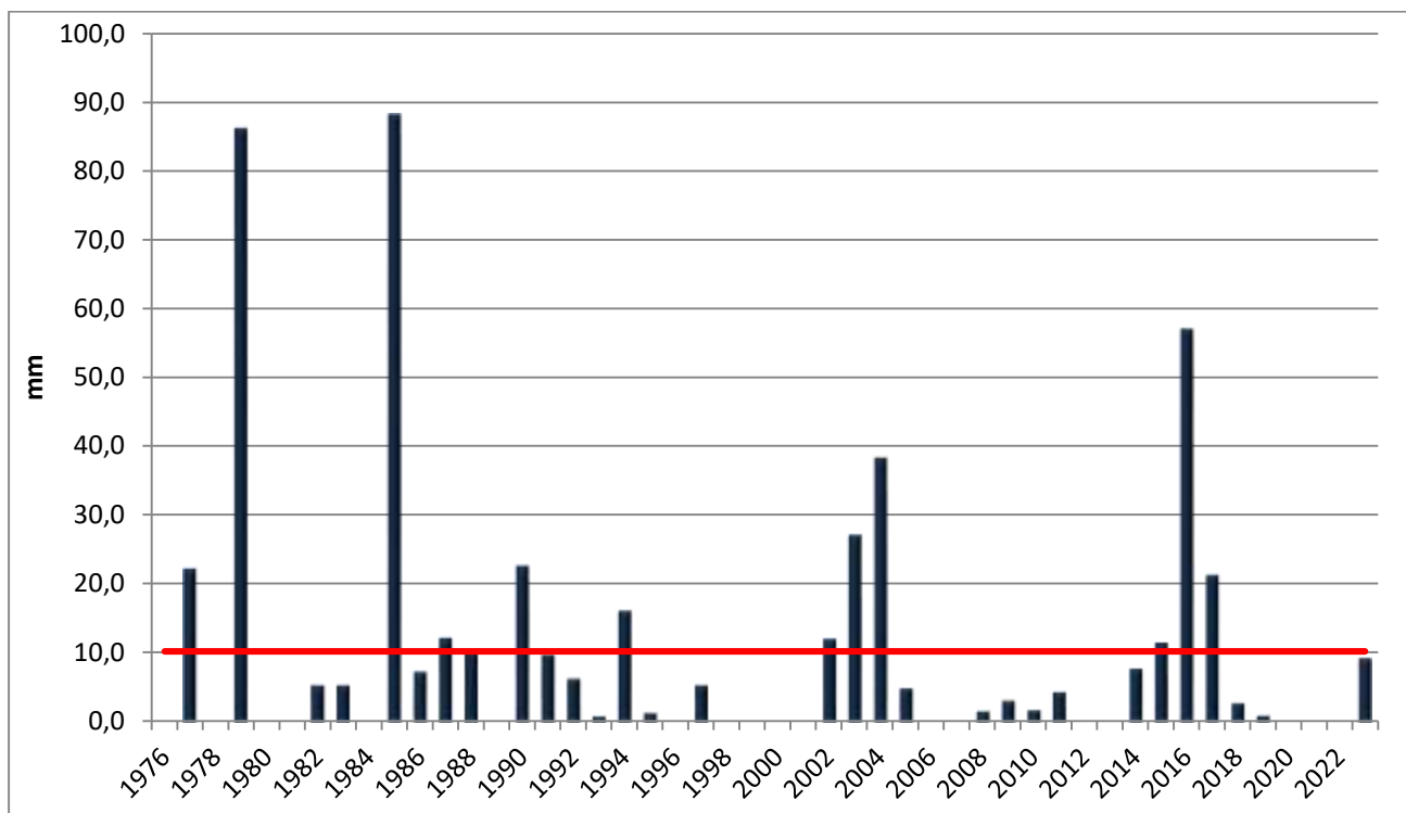
Gráfico 1. Línea roja: Promedio histórico 10.1 mm
